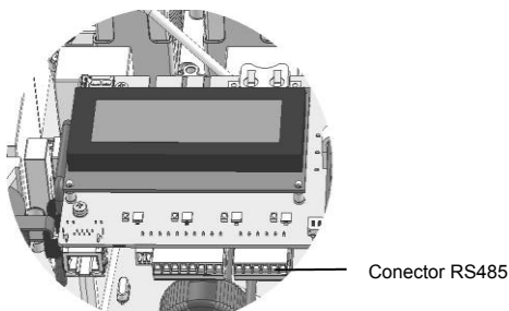
Figura 19. Bloque de terminales RS485
