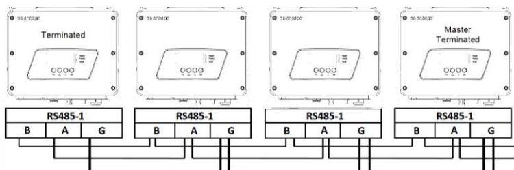
Figura 21. Conectar los inversores en serie
