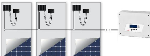
Figura 6. Conexiones de CC del inversor
