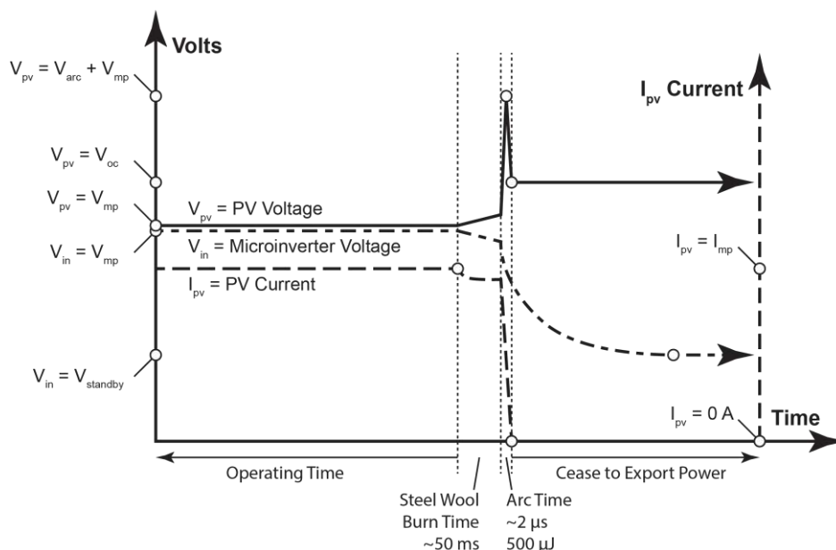
Figuur 5: I-V-curves geven een toelichting op het gedrag van een micro-omvormer tijdens een vlamboog.
